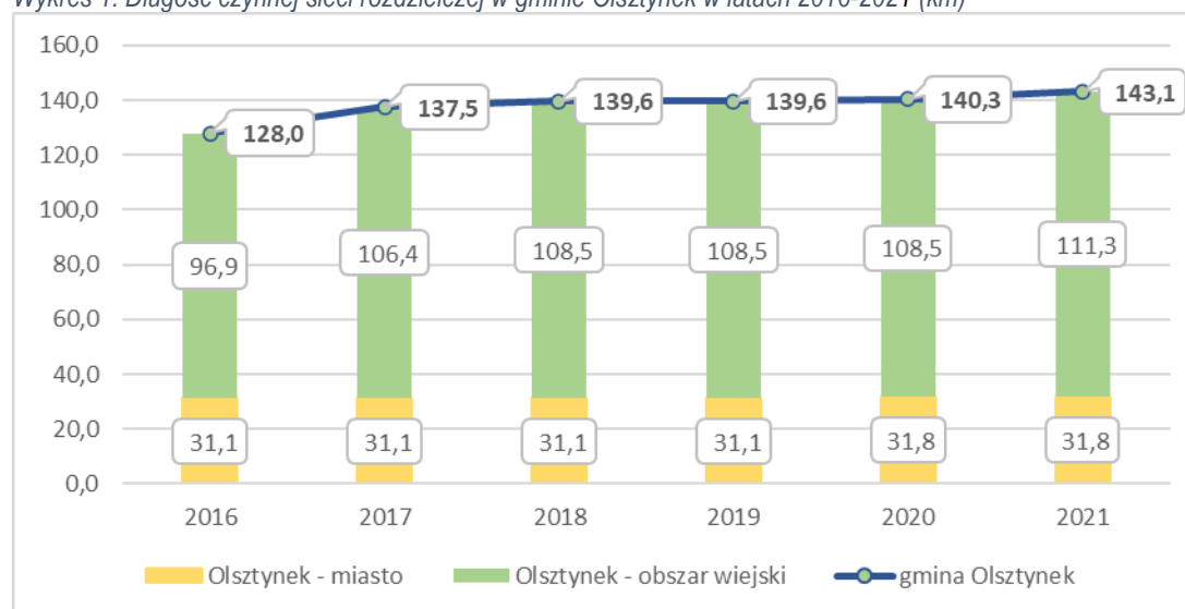
Wykres 1. Długość czynnej sieci rozdzielczej w gminie Olsztynek w latach 2016-2021 (km)
